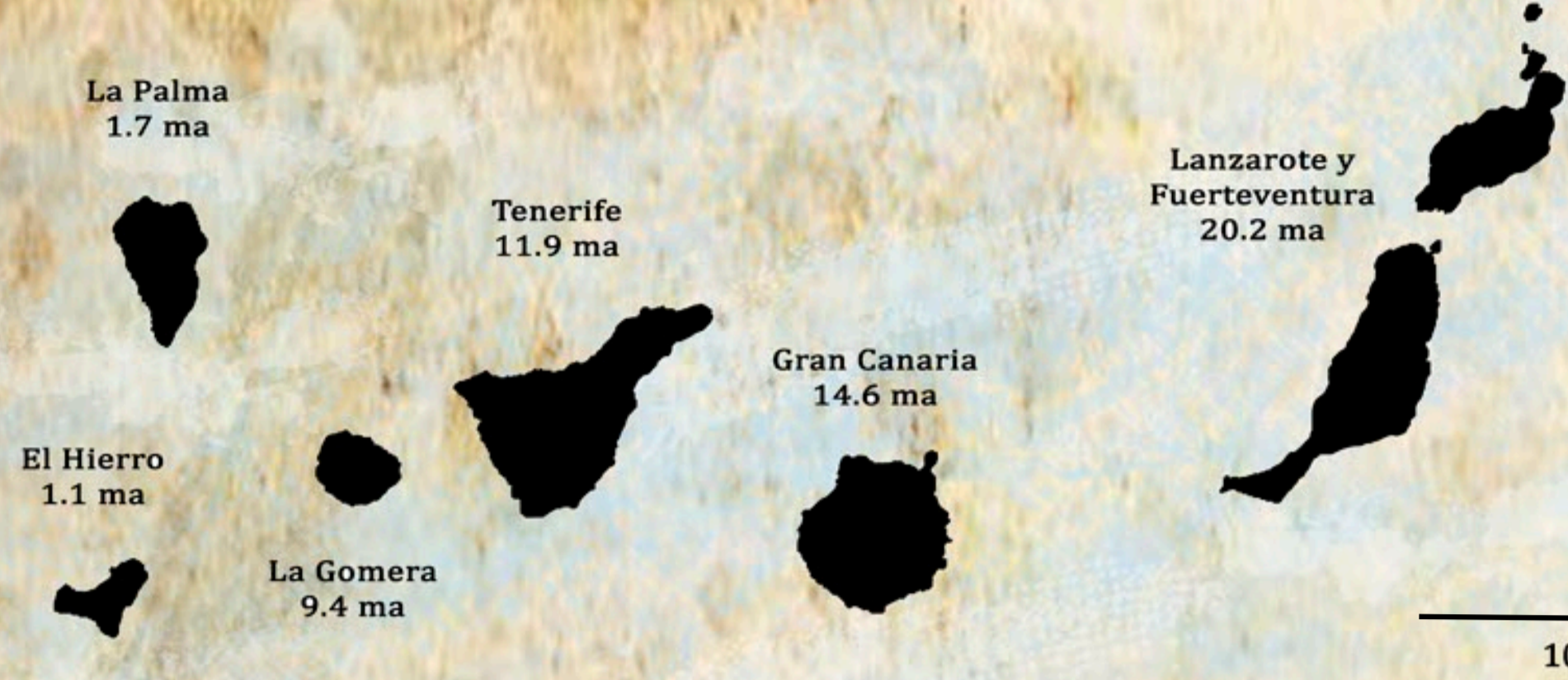
FIGURA 1. Edad de formación de las Islas Canarias.
