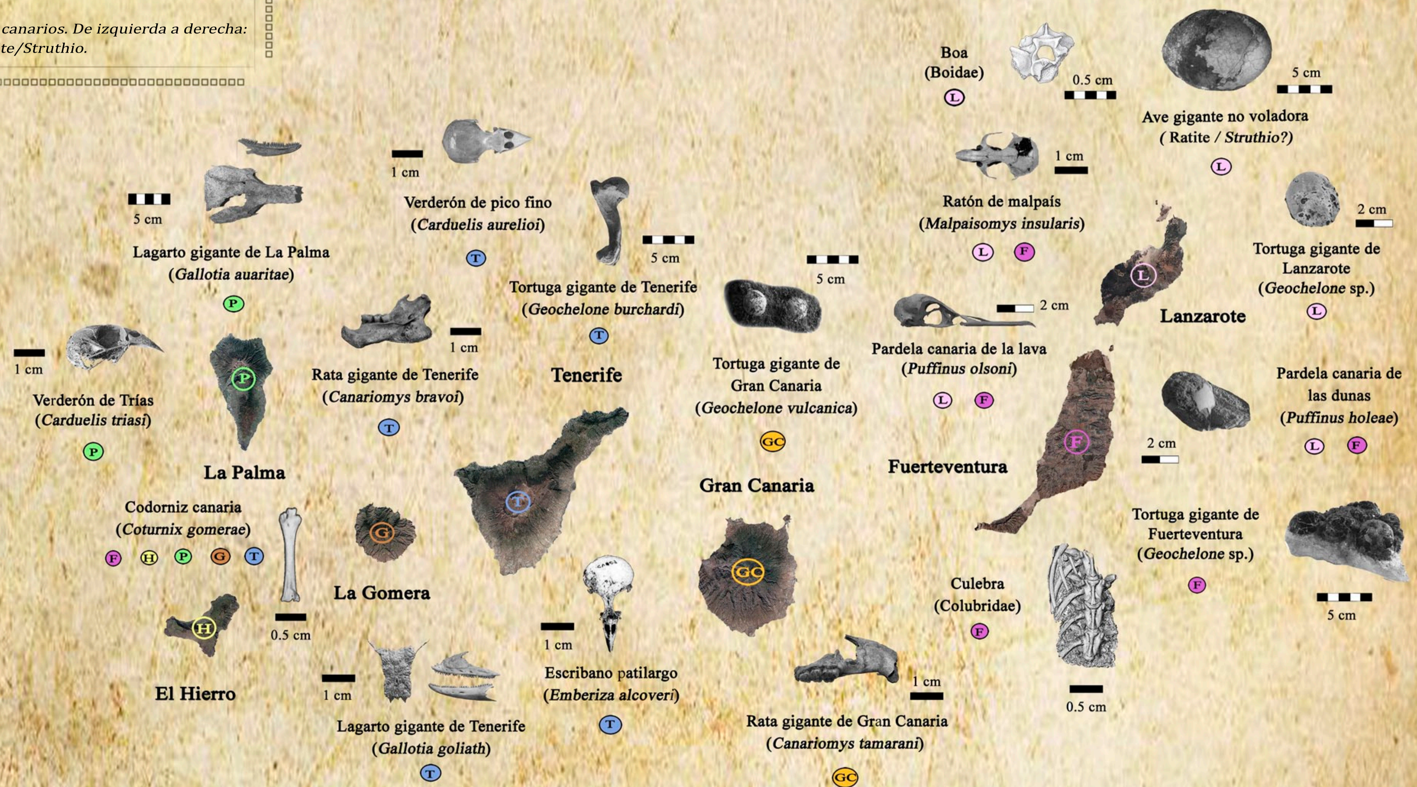
FIGURA 3. Mapa de distribución de los vertebrados fósiles terrestres extintos de las Islas Canarias. Tabla explicativa del mapa anexo con datos del material que se muestra, distribución y edad de la especie.
