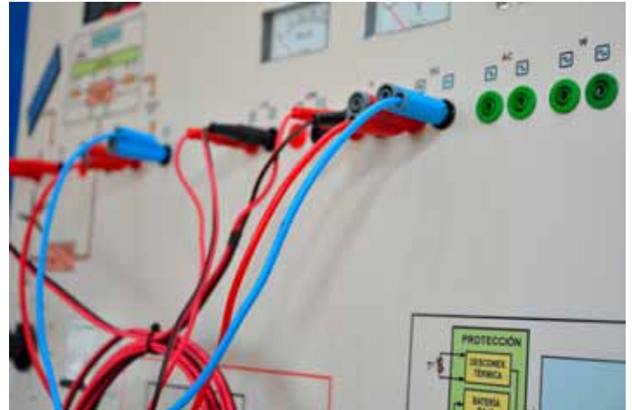
Entrenador modular híbrido fotovoltaica y eólica
